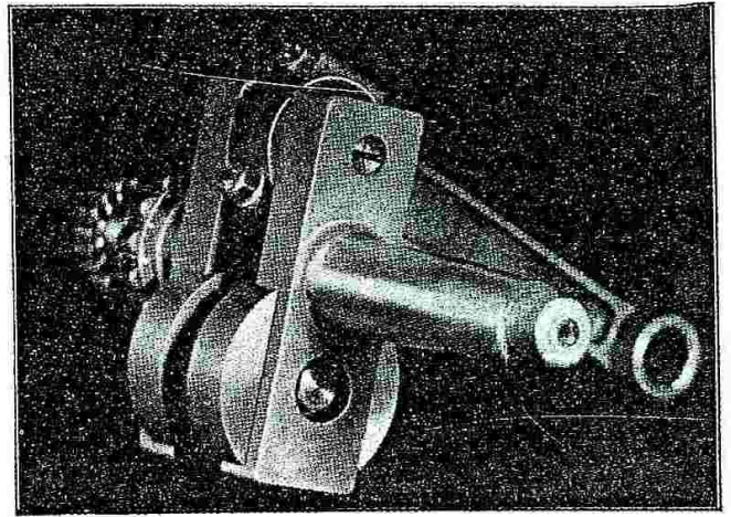
Fig. 57 - Albero a gomito biella visto dal lato volano. Si noti il tappo di ispezione per canale interno dell'olio.
