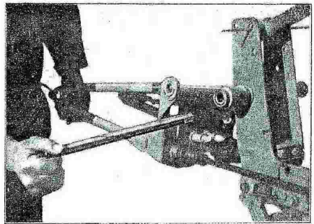
Fig. 28 - Come si leva il forcellone oscillante completo e i tiranti.
