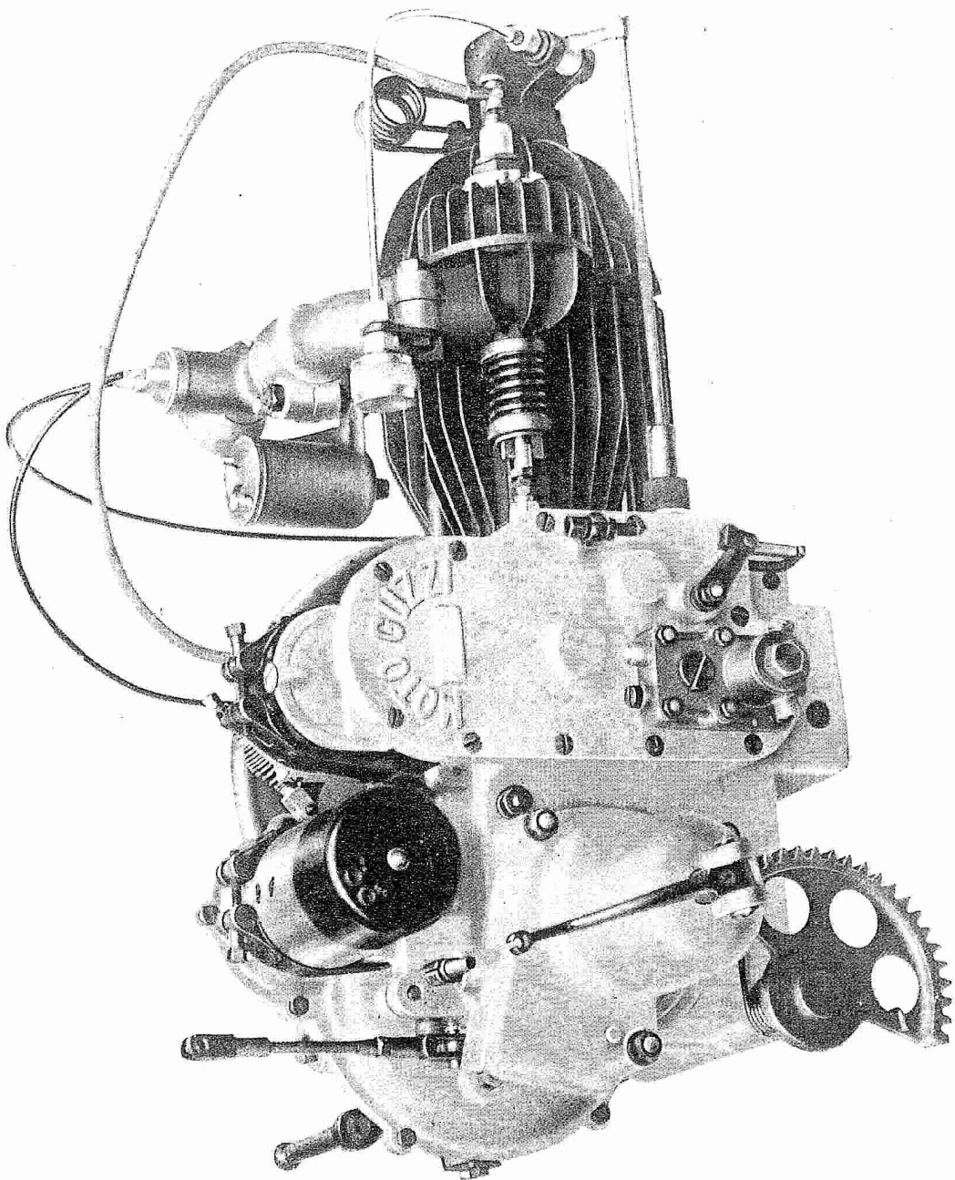
Fig. 1 - Gruppo motore cambio, lato distribuzione
