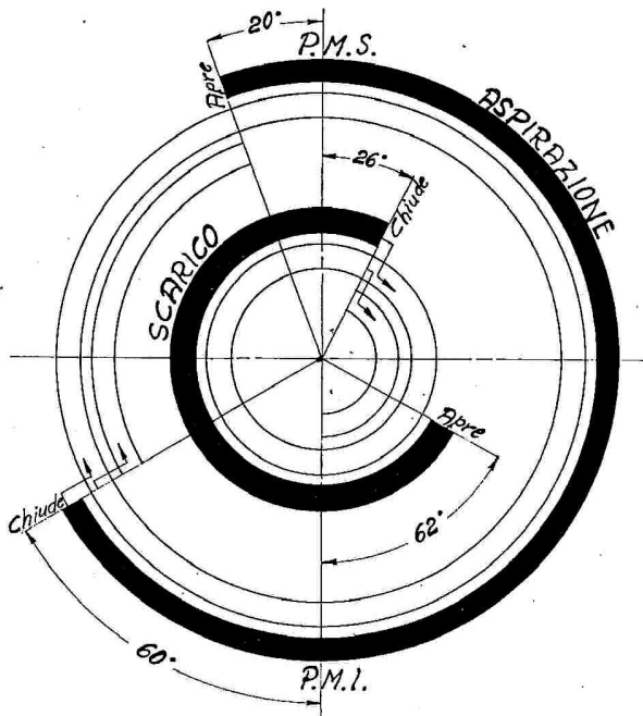
Diagramma angolare di distribuzione riferito all'asse motore
