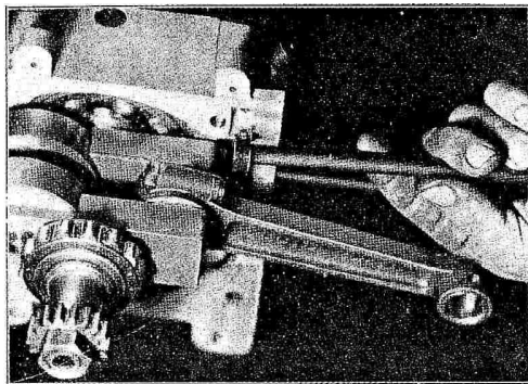
Fig. 75 - Prima di chiudere i due mezzi carter ricordare di piazzare il tirante per fissaggio testa e cilindro.
