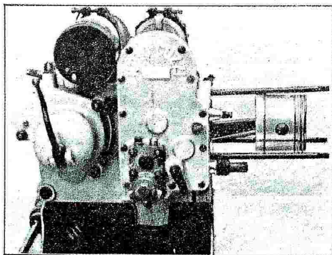
Fig. 38 - Motore senza cilindro e testa.
