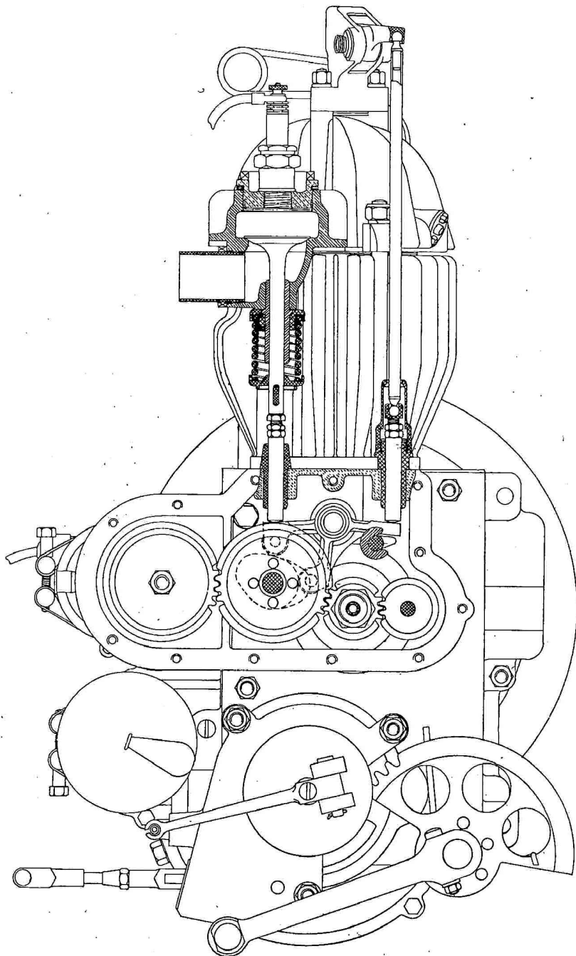
Vista del motore dal lato distribuzione.
