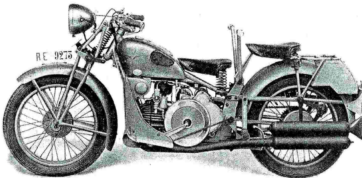
Fig. 11 - Moto "Biposto," lato volante
