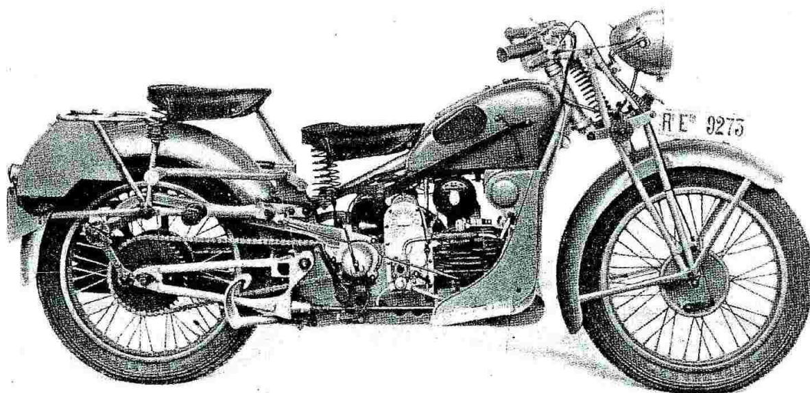
Fig. 12 - Moto "Biposto," lato distribuzione.
