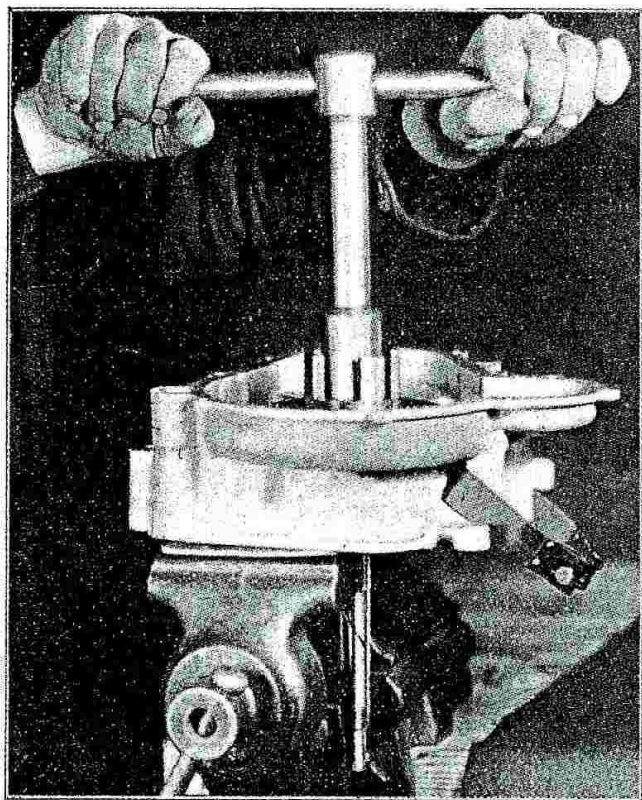
Fig. 50 - Come si prende in morsa l'albero primario del cambio e si smontano il controdado e dado di bloccaggio del corpo frizione fisso (griffa).
