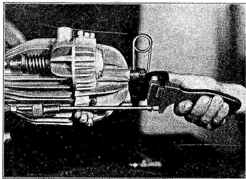
Fig. 76 - Come si monta l'asta di comando per bilancere di scarico.
