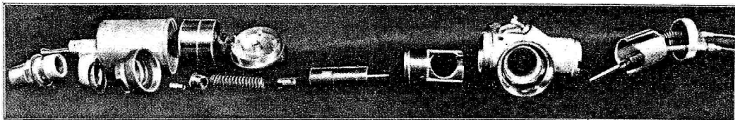
Fig. 67 - Il carburatore smontato.
