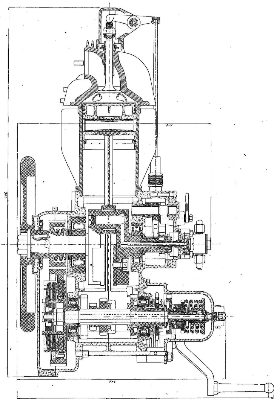
Sezione longitudinale orizzontale del motore.
