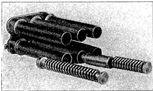
Fig. 84 - Moto biposto. Si notano lo spessore, la molla e la bussoletta di pressione laterali (a sinistra) e centrali.
