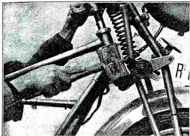
Fig. 29 - Come si sfila il canotto di guida dalla testa di sterzo.
