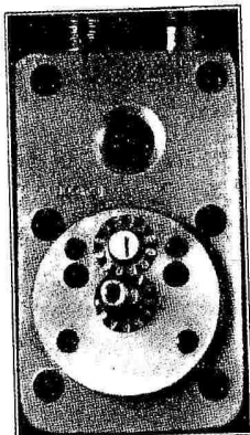
Fig. 71 - Il corpo pompa visto dall'interno. È visibile la pompa di mandata a ingranaggi.
