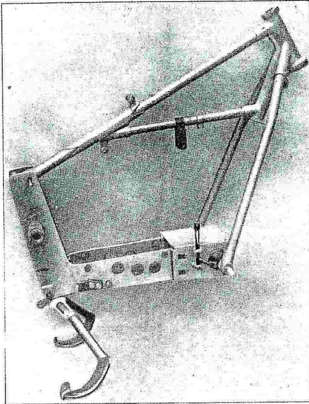
Fig. 31 - Vista del telaio centrale.
