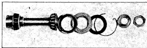
Fig. 87 - Mozzo anteriore. Ordine di montaggio dei vari pezzi.
