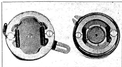
Fig. 89 - Piatto portaceppi posteriore e anteriore.
