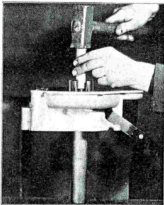
Fig. 51 - Dopo avere infilato sull'albero primario un tubo di ferro, ecco come si sfilare l'albero medesimo.
