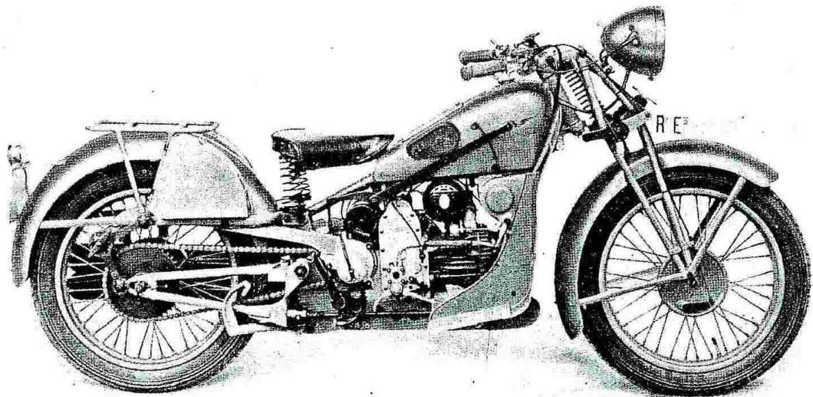
Fig. 8 - Moto "Monoposto", lato distribuzione.
