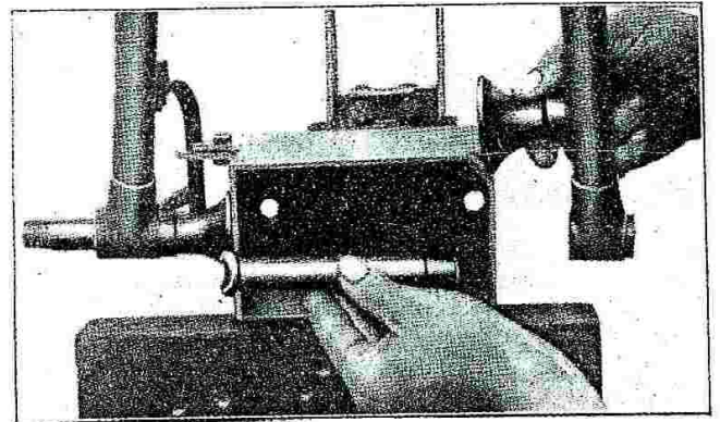
Fig. 32 - Come si levano i due mezzi perni e i rocchetti spessore.
