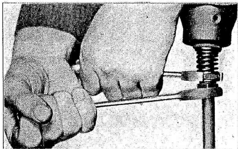
Fig. 85 - Dopo avere leggermente compressa la molla ecco come si serri il morsetto di fissaggio.
