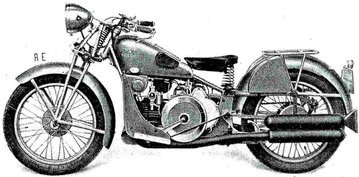
Fig. 7 - Moto "Monoposto", lato volano.
