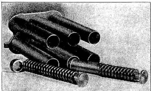
Fig. 83 - Moto monoposto. Si notano la vera spessore, la molla e la bussoletta di pressione laterali (a sinistra) e centrali.
