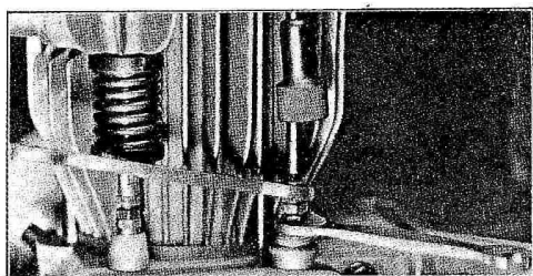
Fig. 77 - Come si regolano le punterie.
