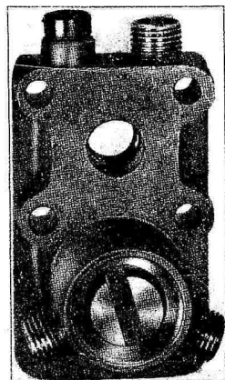
Fig. 72 - Il corpo pompa visto dall'esterno. È visibile la pompa di recupero a palette scorrevoli.
