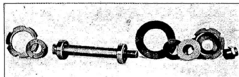
Fig. 88 - Mozzo posteriore. Ordine di montaggio dei vari pezzi.
