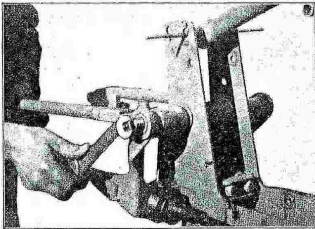
Fig. 26 - Come si leva il perno principale del forcellone oscillante.
