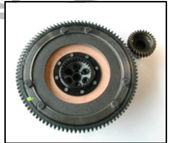
frizione mono/mono clutch
