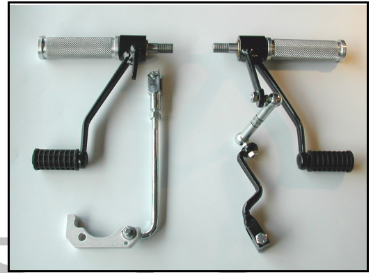
pedane arretrate Agostini/Agostini rear sets
