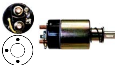
131799# Solenoid
