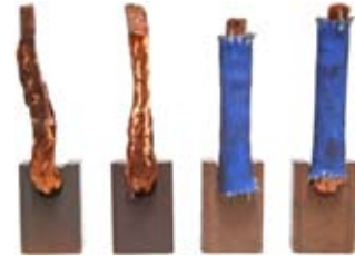
140347 Brush Set Replacing: TAJ203 12 V., L. 17.00, Th. 6.80, H. 12.00
