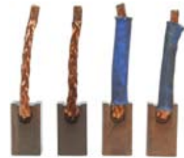
140349 Brush Set Replacing: TAJ209 12 V., L. 17.00, Th. 7.00, H. 10.00
