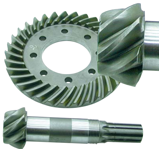
Beispiel einer Kardanübersetzung von einer SP1000 zum Tellerradsatz 7/33 im Verhältnis von 1:4.714
