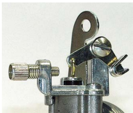
Detailbild der Gaszugsteuerung am SHA Vergaser.
