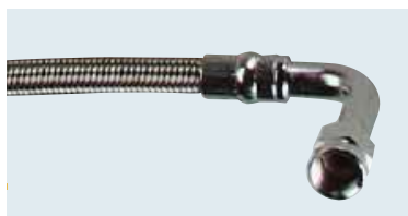
Leitung-Kit Typ 1= Stahlflexleitung und Anschlüsse aus Stahl
