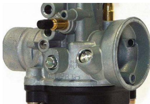
Leerlauf- und Gemischeinstellung
