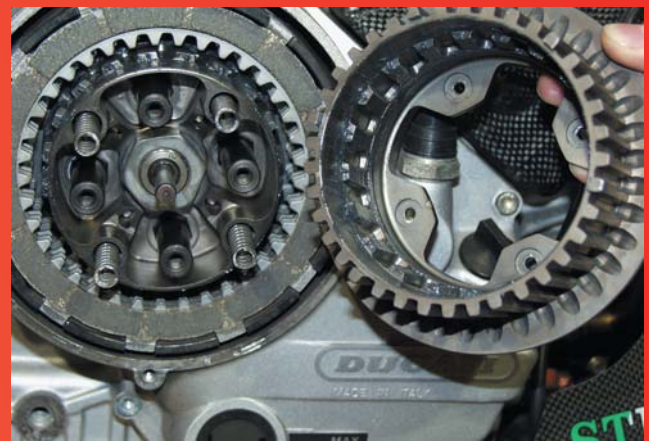
Innenansicht der eingebauten Adler (APTC) Antihoppingkupplung.
