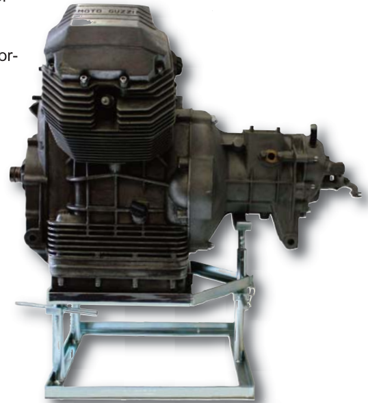
Der Motorständer im Einsatz
