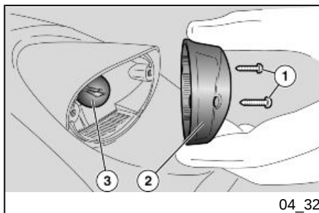
Grupo óptico trasero (04_32, 04_33, 04_34)
