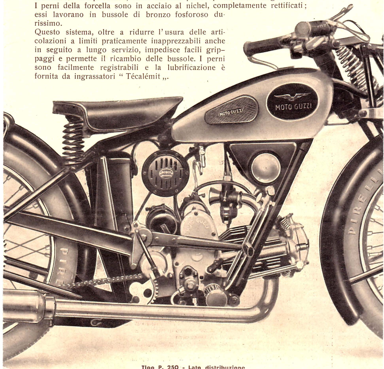
Tipo P. 250 - Lato distribuzione
