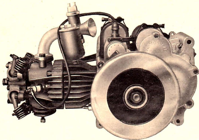
Il motore visto dal lato del volano
