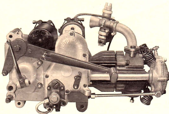
Il motore visto dal lato della distribuzione
