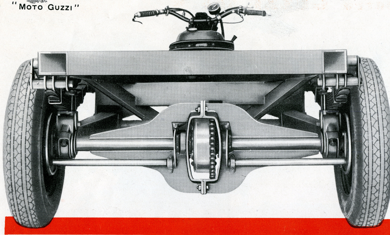
SOSPENSIONE - DIFFERENZIALI E FRENI POSTERIORI
