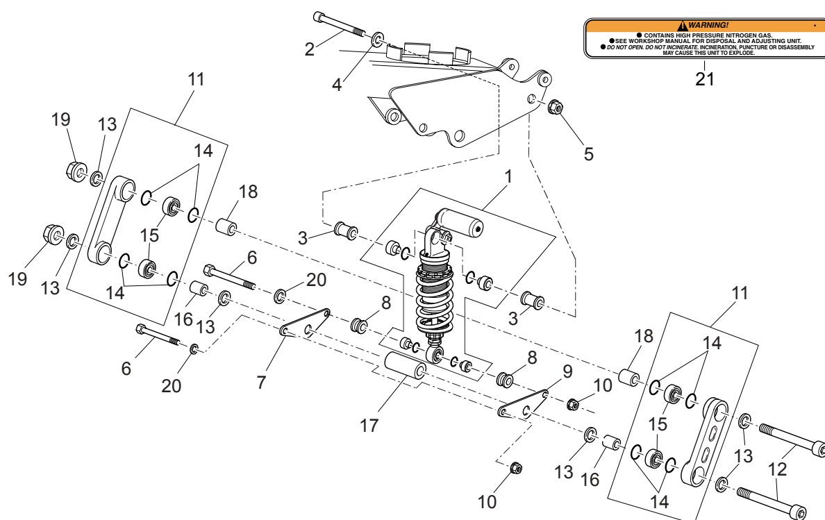
TAVOLA 32 - BIELLETTA E AMMORTIZZATORE POST.
