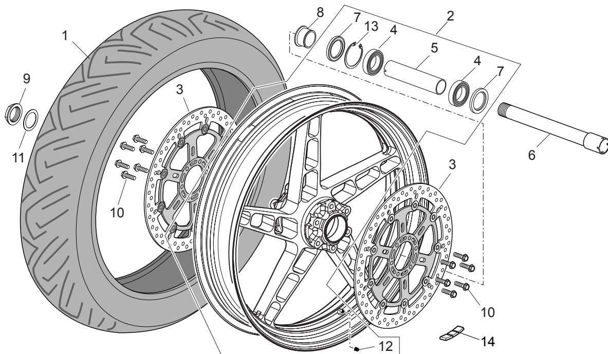
TAVOLA 33 - RUOTA ANTERIORE
