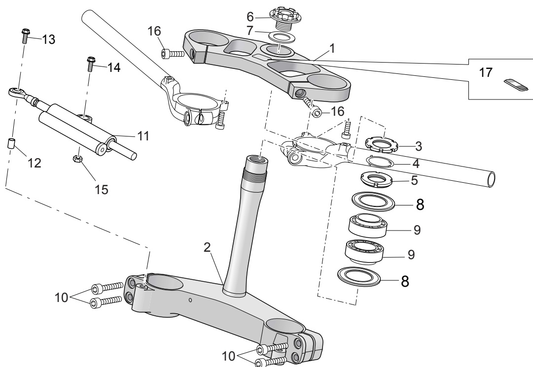
TAVOLA 29 - STERZO
