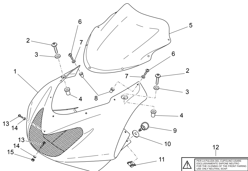
TAVOLA 25 - CUPOLINO
