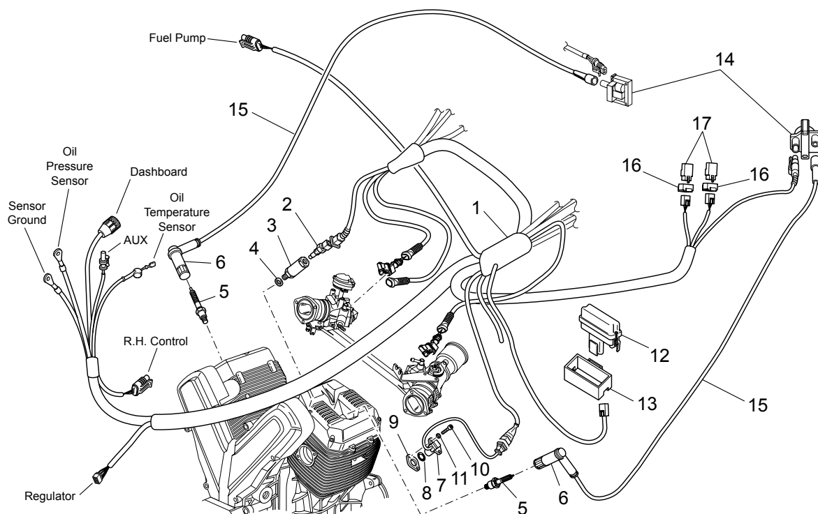
TAVOLA 44 - IMPIANTO ELETTRICO I
