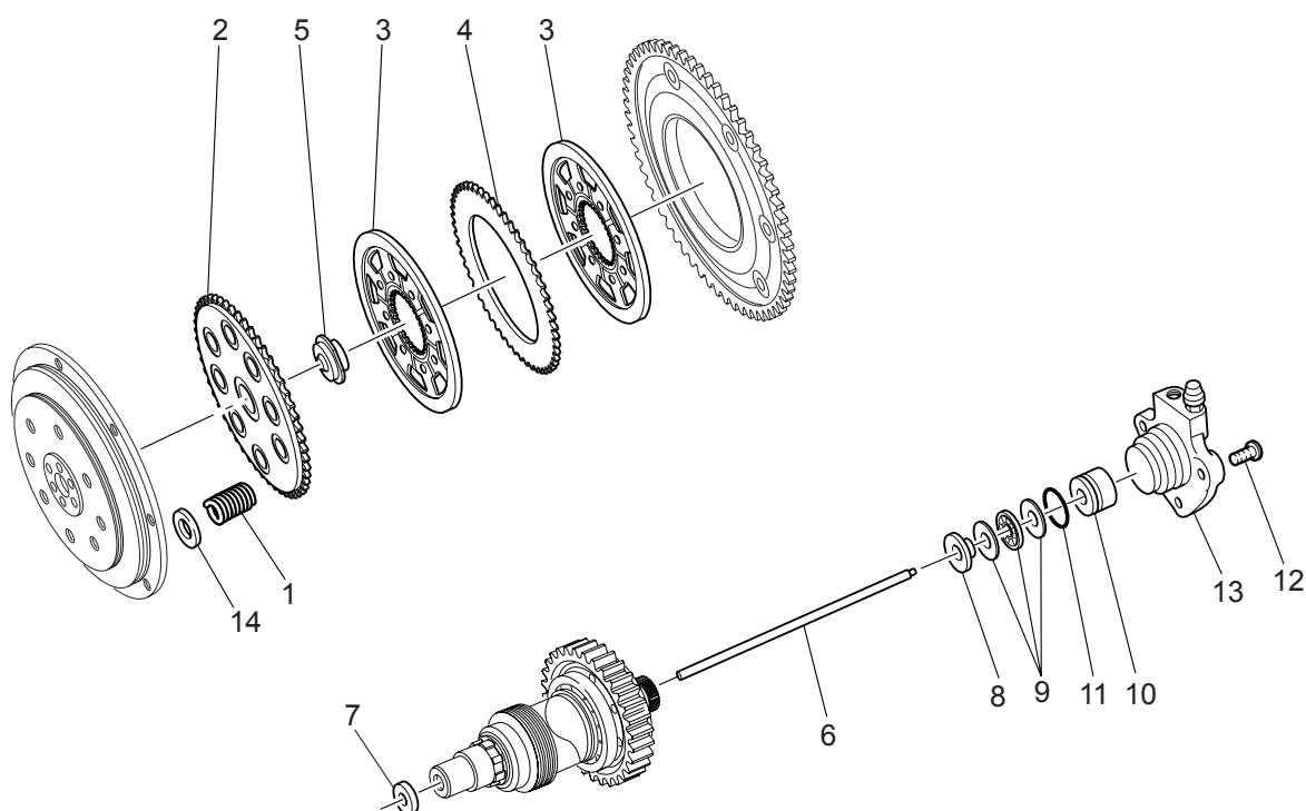
TAVOLA 13 - FRIZIONE
