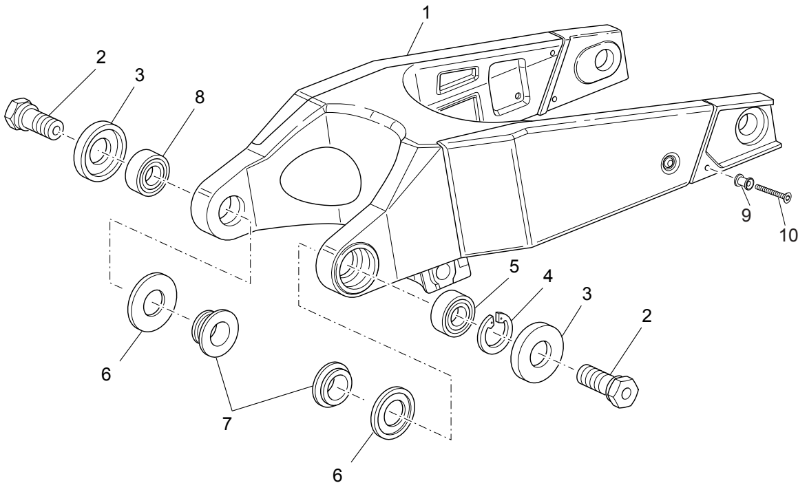
TAVOLA 31 - FORCELLONE
