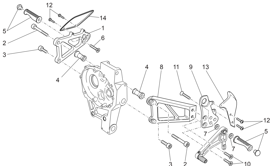
TAVOLA 23 - PEDANE
