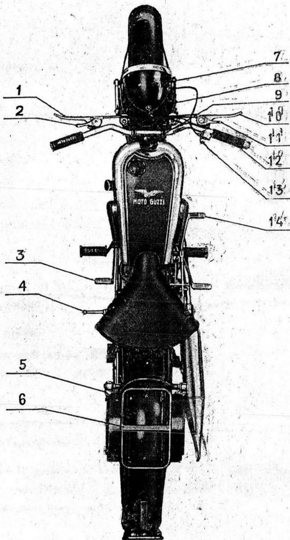
Fig. 3 — Motociclo AIRONE (comandi e accessori)
