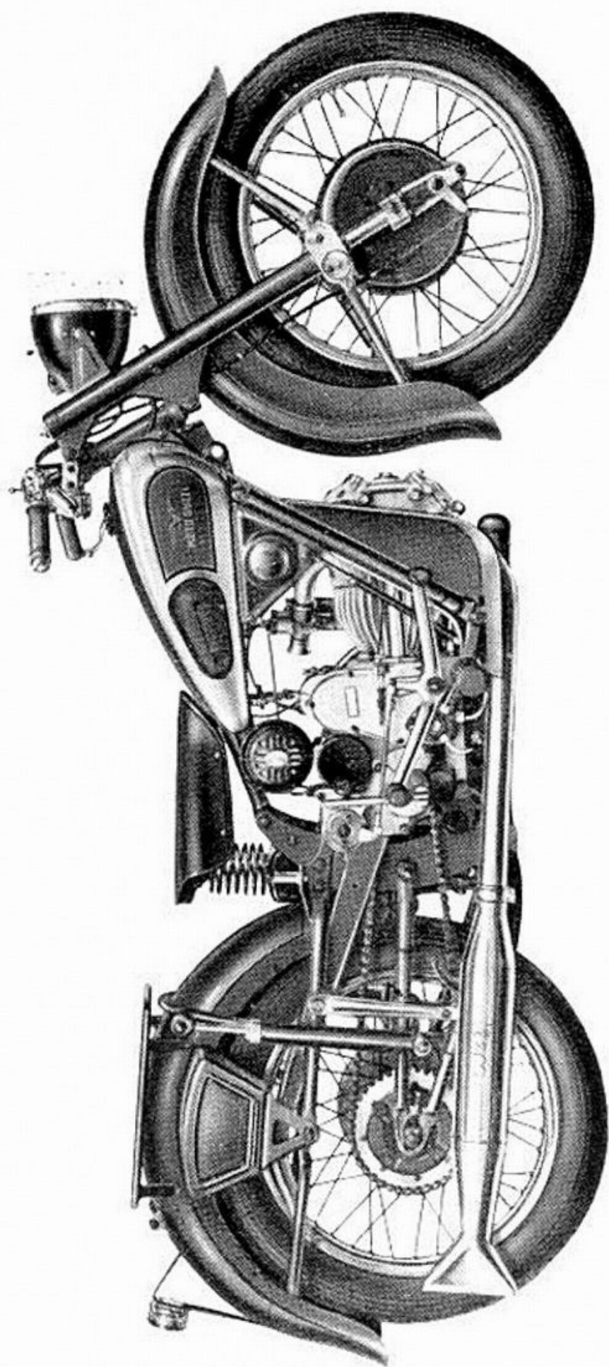
Fig. 2 - Motociclo Astore (lato distribuzione)
