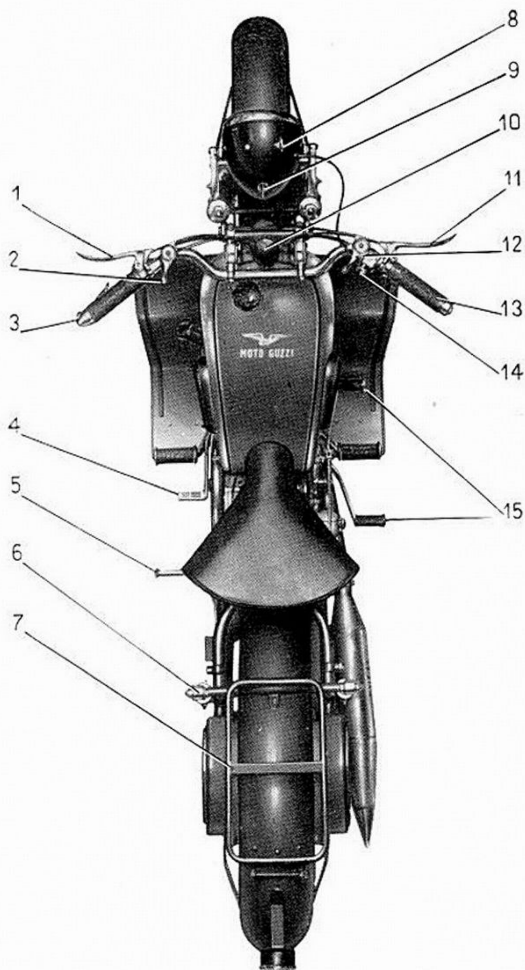
Fig. 3 - Motociclo Astore (comandi ed accessori)
